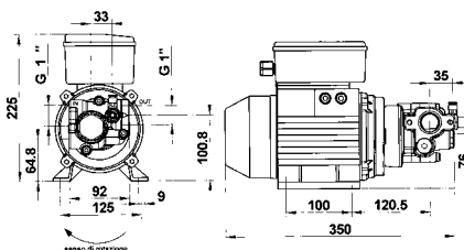
Viscomat 350/2 Viscomat 230/3
